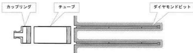
深あな穿孔の方法
